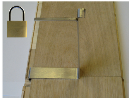
7. Rückwärts Verlegung Feder positionieren
