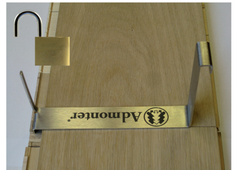
8. Rückwärts Verlegung verriegeln
